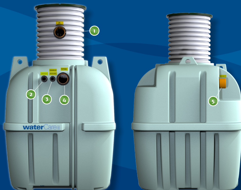
4 m³ husanlæg med oversigt over tilslutninger. Samme opbygning er gældende for de andre tankstørrelser
