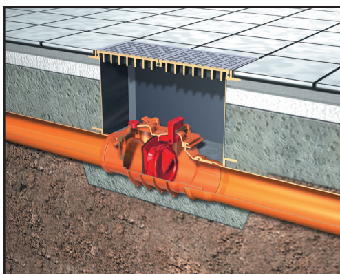
Monteres vandret i gulv, ved hjælp af et firkantet forhøjerstykke og et dæksel af plast.
