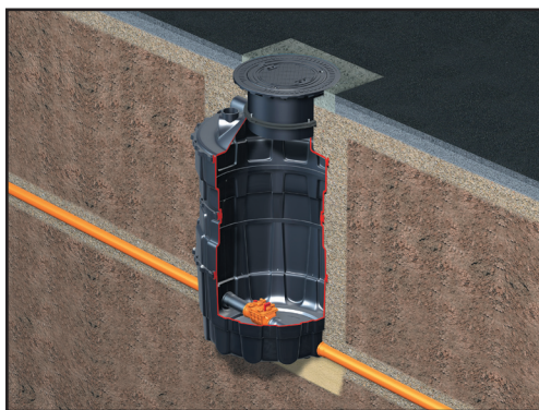
Monteres vandret i eks. Ø1000 plast brønd
