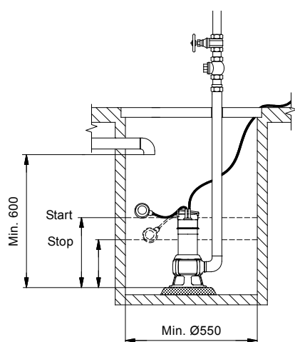
Fig. 27 Min. brøndmål, Unilift AP35B
