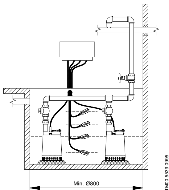
Fig. 18 2-pumpeinstallation med fire svømmerafbrydere
