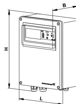
Fig. 43 Målkitse, styreskab
