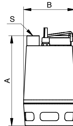
Fig. 21 Pumpemål
