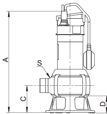
Fig. 26 Pumpemål
