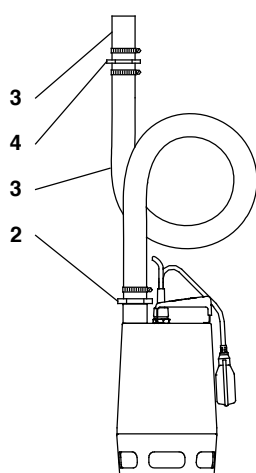
Fig. 46 Unilift-slangetilslutning
