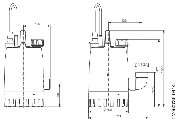
Fig. 6 Pumpemål
