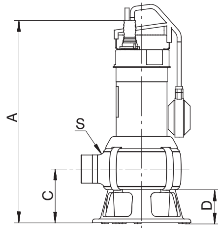
Fig. 37 Pumpemål
