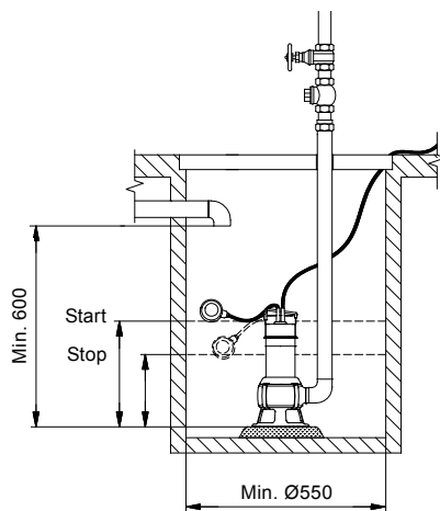
Fig. 38 Min. brøndmål, Unilift AP50B
