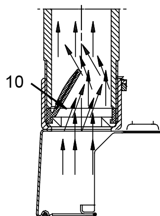
Fig. 48 Funktionsskitse af kontraventil i Unilift-pumpeafgang
