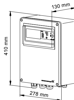
Fig. 45 Målskitse, styreskab
