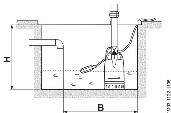
Fig. 4 Min. brøndmål, Unilift CC
