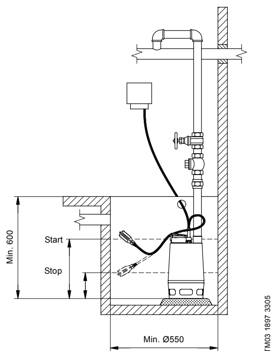
Fig. 33 1-pumpeinstallation med svømmerafbryder
