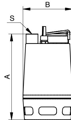
Fig. 32 Pumpemål
