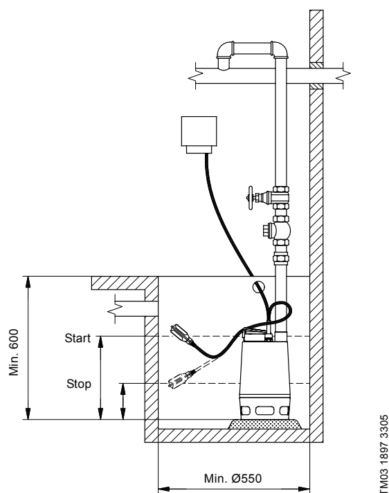
Fig. 22 1-pumpeinstallation med svømmerafbryder
