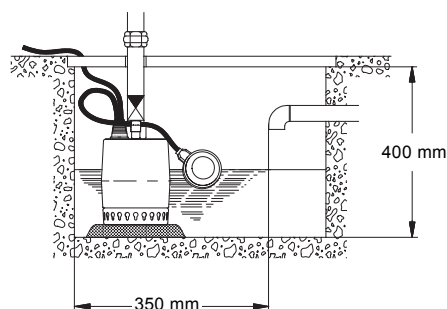
Fig. 8 Min. brøndmål, Unilift KP-A
