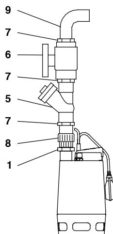
Fig. 47 Unilift-rørtilslutning, afspærringsventil og kontraventil
