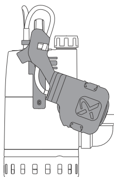
Fig. 5 Unilift CC med niveaupippe monteret
