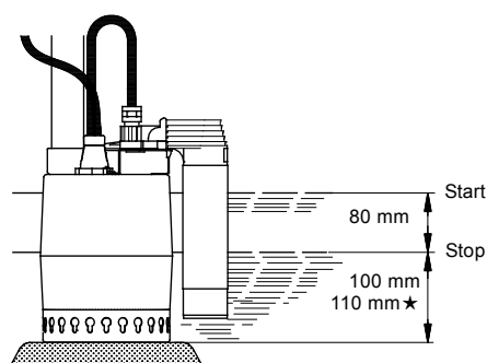
Fig. 12 Start/stop-niveauer for Unilift KP AV
