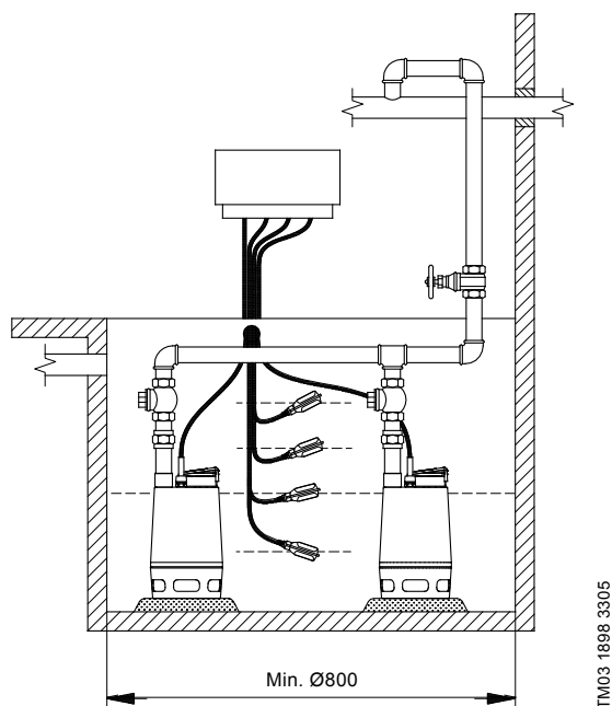
Fig. 23 2-pumpeinstallation med fire svømmerafbrydere
