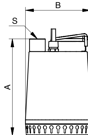
Fig. 16 Pumpemål
