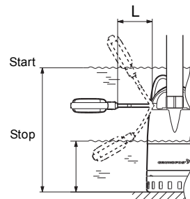
Fig. 3 Start-/stopniveau, Unilift CC
