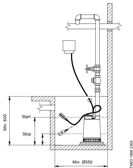
Fig. 17 1-pumpeinstallation med svømmerafbryder
