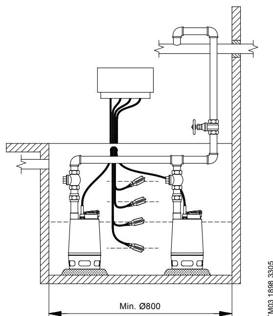
Fig. 34 2-pumpeinstallation med fire svømmerafbrydere
