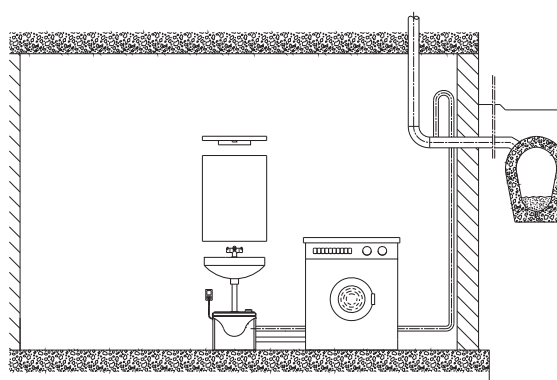
Fig. 3 Installationseksempel
