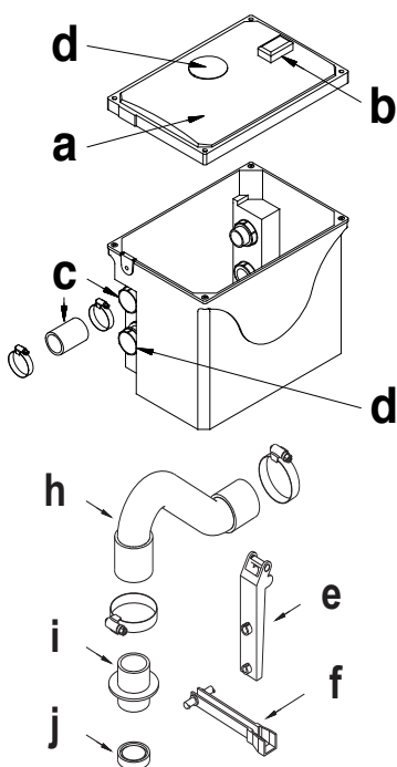
Fig. 1 Komponentliste Liftaway C 40-1
