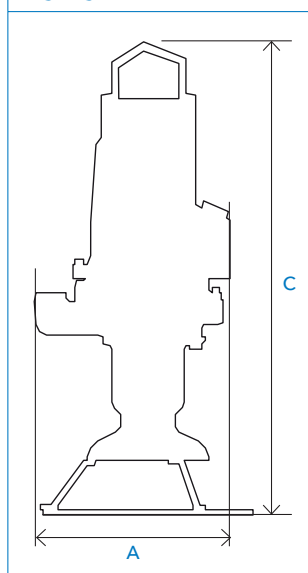
Tegning: MF 3068
