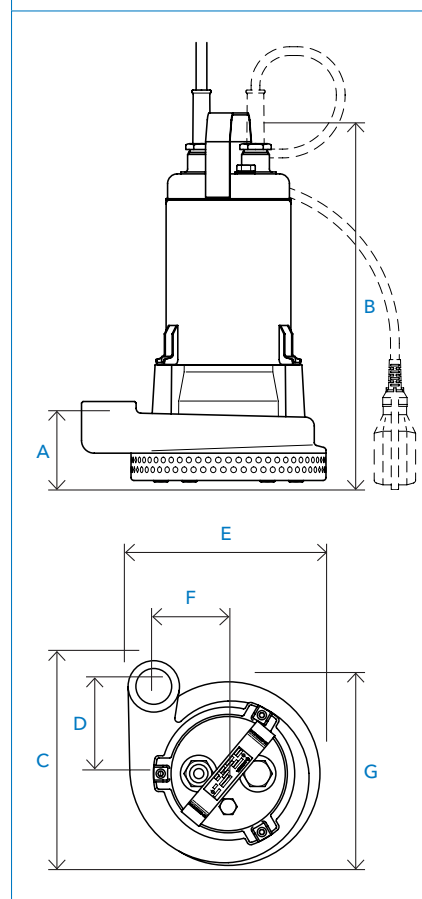
Tegning
