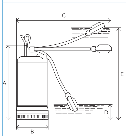
Tegning: SX 5-15
