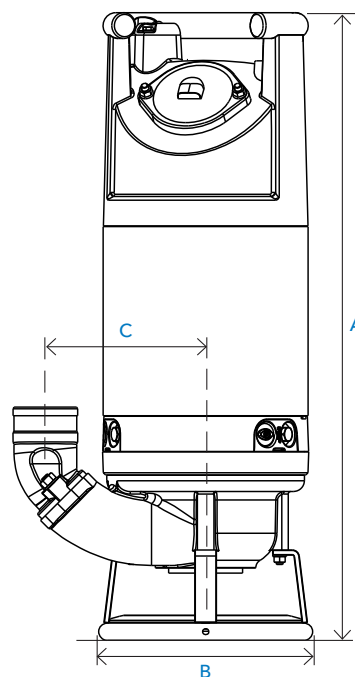
Tegning: DS 2620
