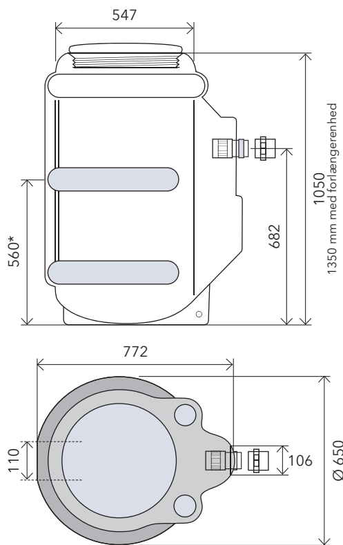
Tegning: Micro 5G/7G
