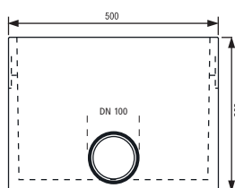
Udløbskasse inkl. galvaniseret slamspand
