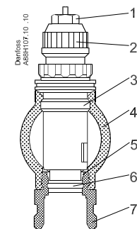
Returmanifold med forindstillingsventil
