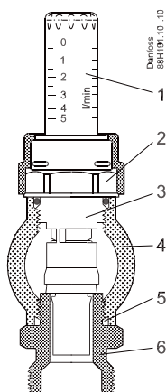
Fremløbsmanifold med flowmeter
