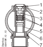
Fremløbsmanifold uden flowmeter
