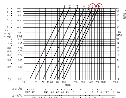
Manifold uden flowmeter
