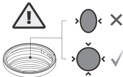
Fig. 19 Oval brønd efter komprimering
