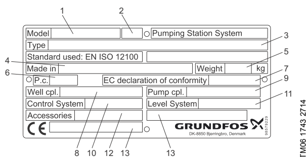
Fig. 2 Typeskilt, PS.S
