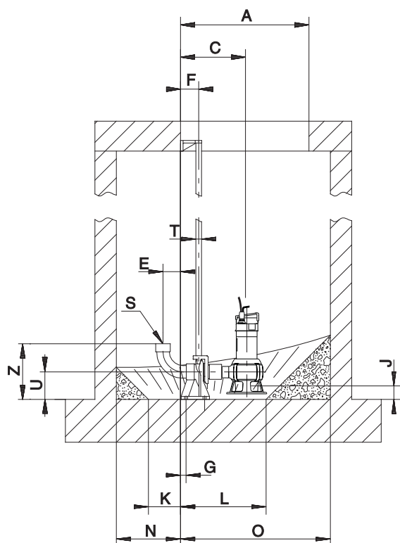
Fig. 39 Målsskitse, 1-pumpeinstallation på autokoblingssystem
