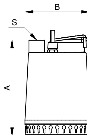
Fig. 16 Pumpemål
