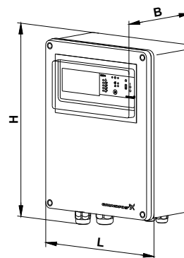
Fig. 43 Målkitse, styreskab
