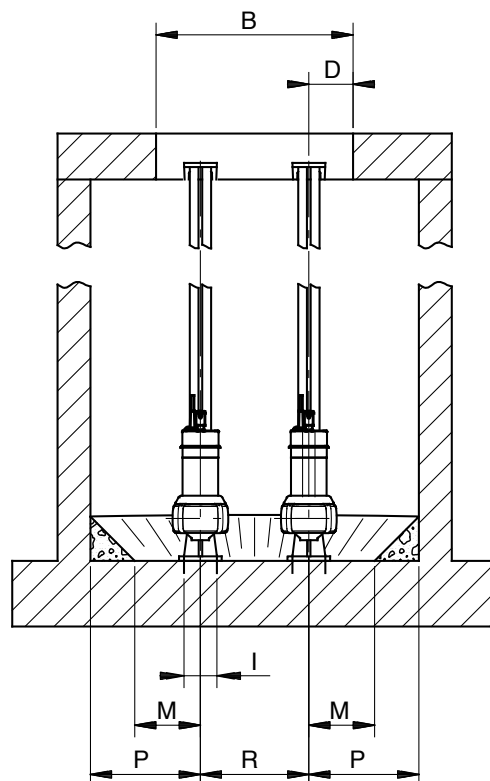
Fig. 40 Målsskitse, 2-pumpeinstallation på autokoblingssystem
