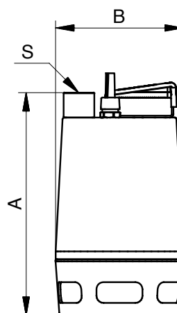
Fig. 32 Pumpemål
