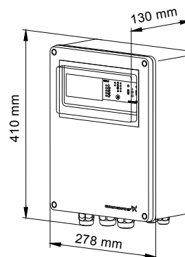
Fig. 45 Målskitse, styreskab
