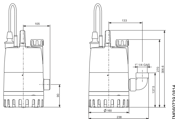
Fig. 6 Pumpemål
