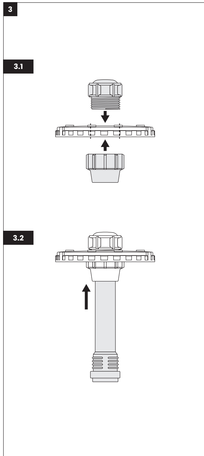
Bild 3: Montera ändpluggen (5) i hålet och fixera med ändpluggsskruven (4) så att muffändan pekar in i tanken (bild 3.1). Tryck ner skyddsroret (3) i botten av ändpluggen (5) (bild 3.2).
