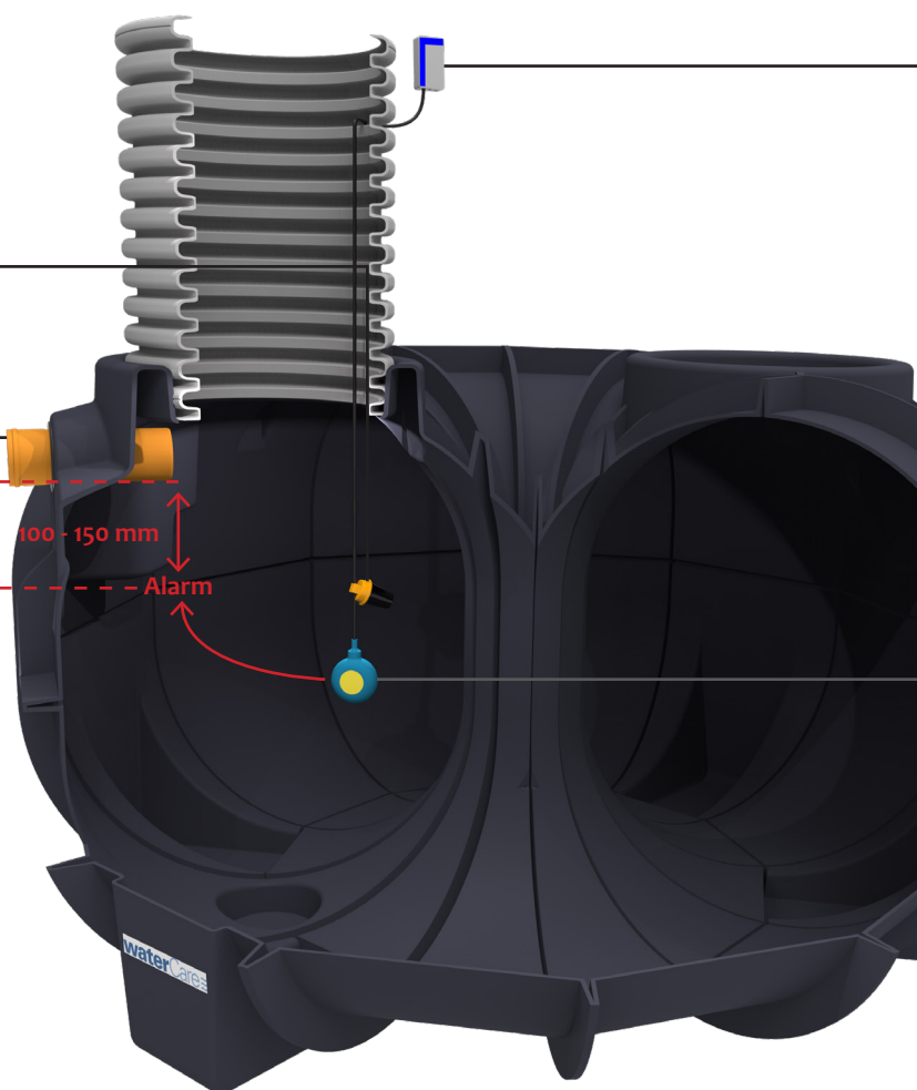
Eksempel på VA-alarm monteret i WaterCare 3.300 L samletank
