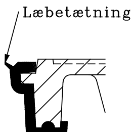
Skitse af pakning.
