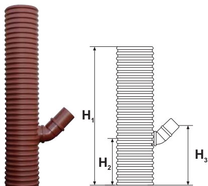
PP Rendestensbrønd med vandlås
