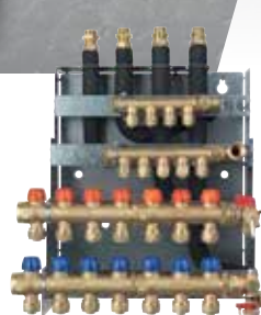
Wavin bundmodul med- og uden isoleringsskåle
