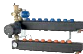
Wavin parallelshunt med- og uden isoleringsskåle
