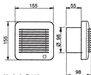
Murhul: Ø 110 mm EDM 100 VM. Rudehul: Ø106 mm
