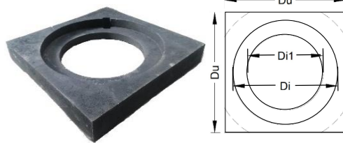
Firkantkarm til Ø315 mm dæksel
