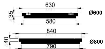
Ø600 / Ø800 karm
