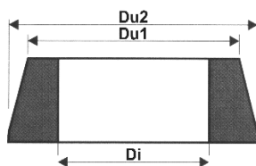
Kegle Ø315/425
