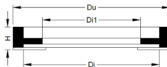
Dæksel m/ karm Ø600 / Ø800 mm består af en topring med fals og et dæksel
